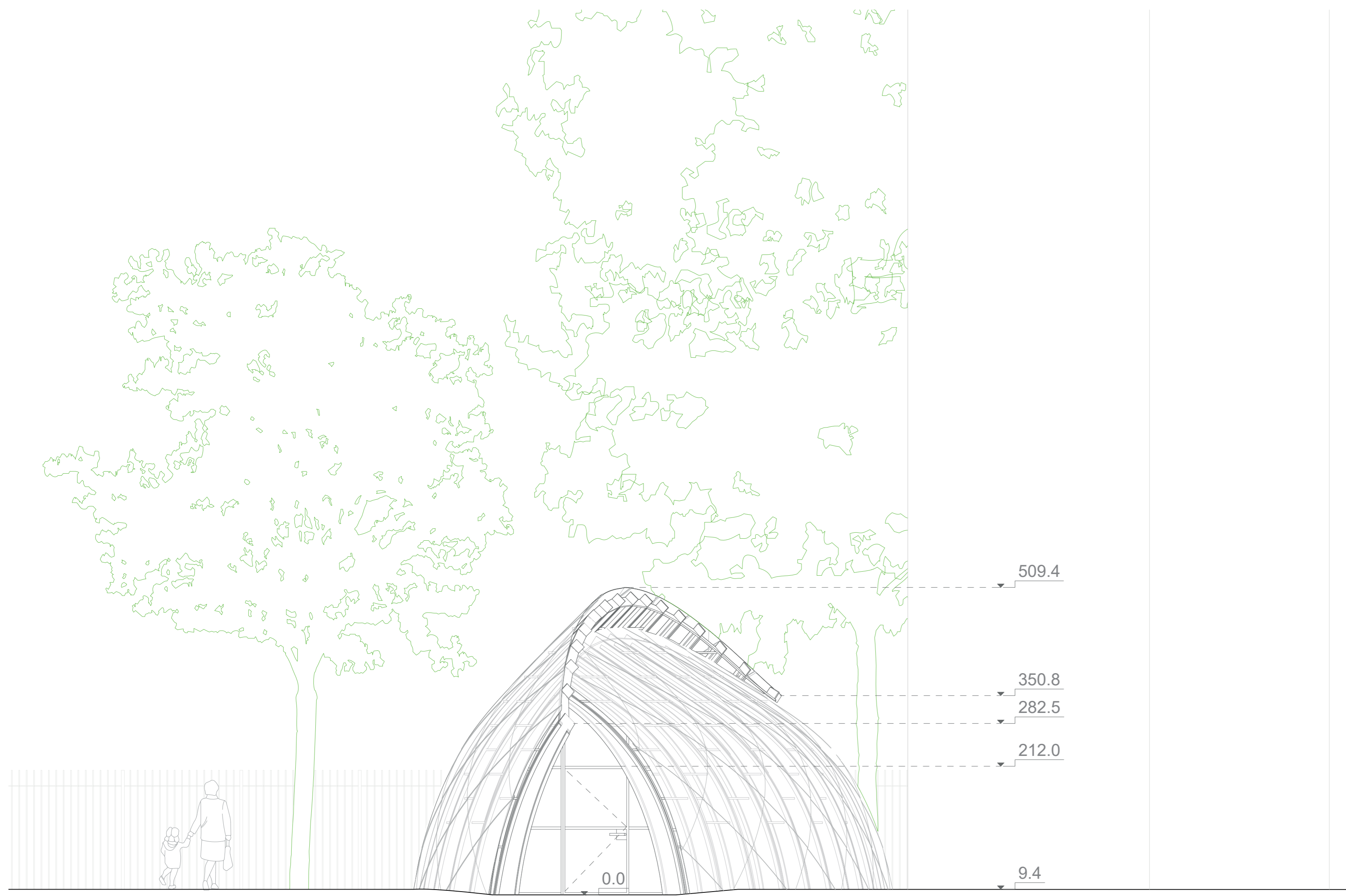
ELEVATION SW
